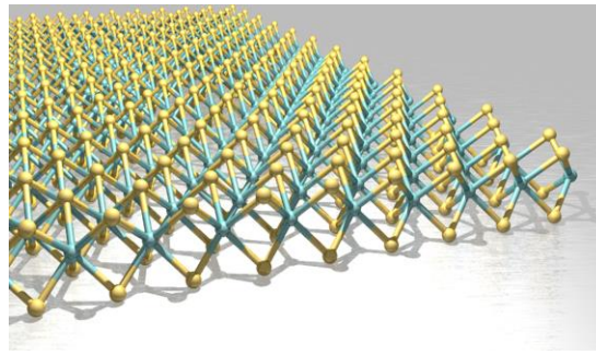
図1 3原子厚(原子3個分の厚さ)の半導体材料である遷移金属ダイカルコゲナイド原子層の模式図。青色が遷移金属原子、黄色がカルコゲン原子に対応する。
